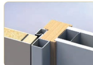
Bâti métallique de réhabilitation sur huisserie bois résineux ou exotique.
